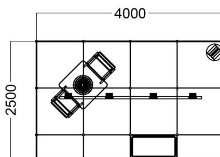
Beispiel Grundriss / example of plan 10 m 2
